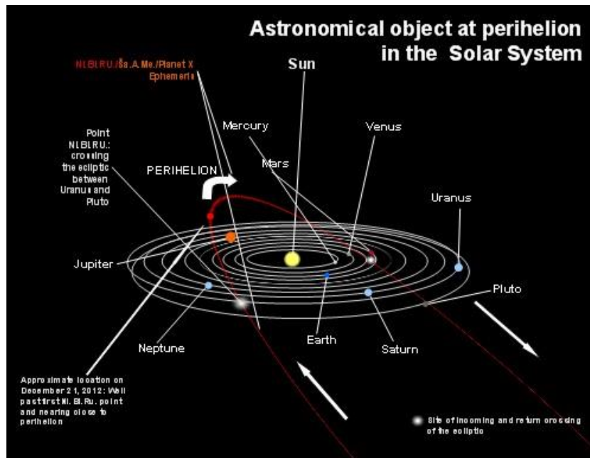
Figura 1-4A. La línea roja indica la supuesta órbita de Ša.A.M.e cuando entra y sale de nuestro sistema solar. El planeta rojo en la línea es la posición estimada de Ša.A.M.e/Nibiru, el 21 de diciembre de 2012, de acuerdo con LPG-C.
