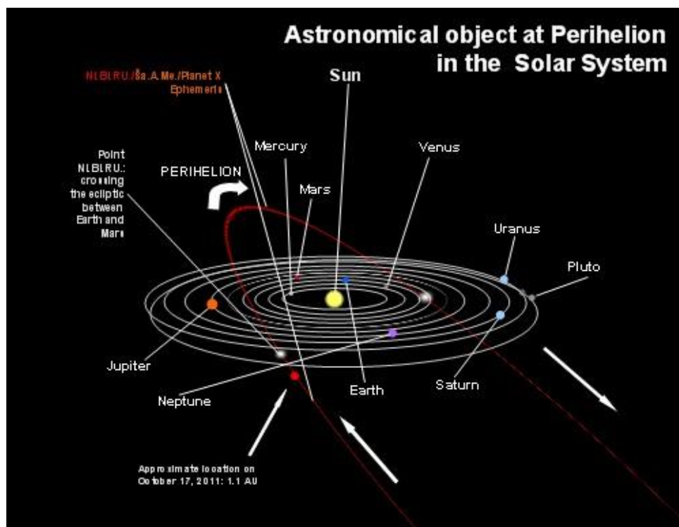
Figura 1-4. La línea roja indica la supuesta órbita de Ša.A.M.e cuando entra y sale de nuestro sistema solar. El planeta rojo en la línea es la posición de Ša.A.M.e/Nibiru el 17 de octubre de 2011, entonces aprox. a 1UA de la Tierra - más exactamente 93,000.000 millas + un extra 17,000-18,000 millas más, de acuerdo con LPG-C.
