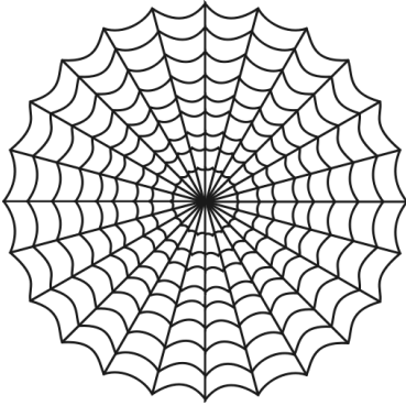
Figura 2-2. Múltiples universos, conectados como una tela de araña.
