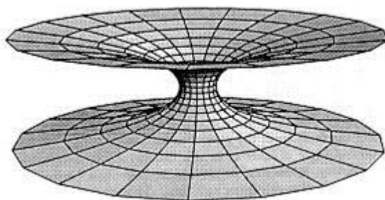
Fig 2-6. Puente de Einstein-Rosen.
