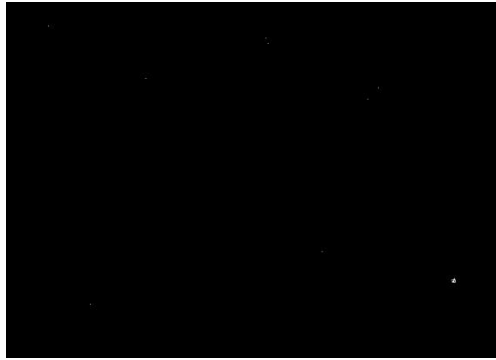
Figure 1: A dying universe, more or less depleted of light Figura 1: Un universo de morir, más o menos agotado de luz
